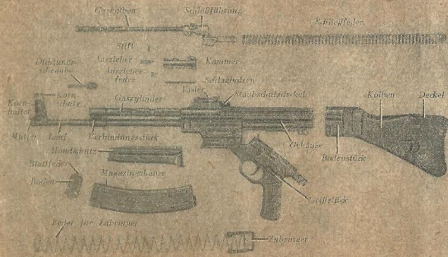
Bild 2: SIG 44 und Magazin, zum Reinigen auseinandergenommen
